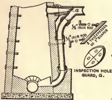
FIG. 8. DROP MANHOLE.
